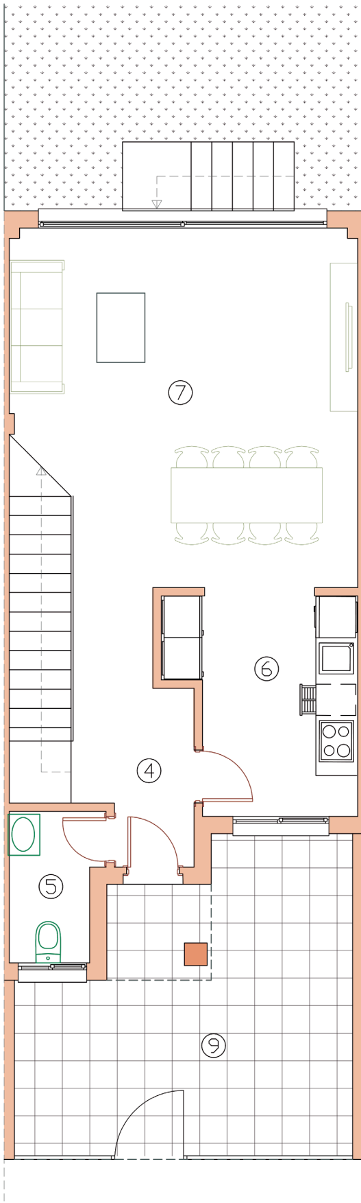
PLANTA BAJA
